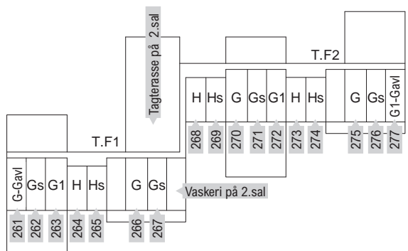
2. salsplan
