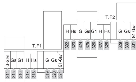
5. salsplan
